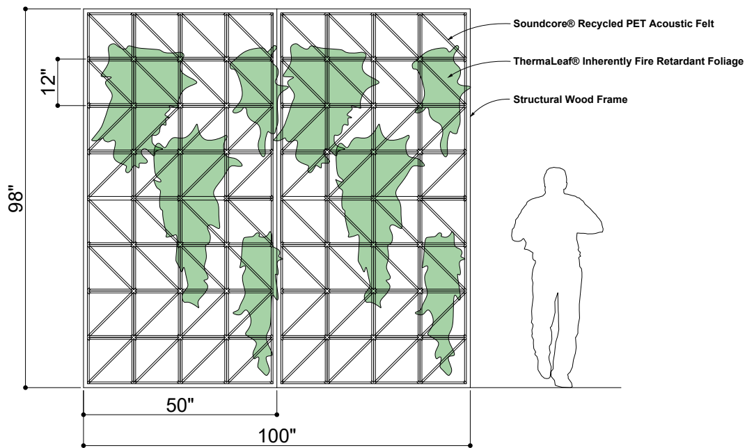
② ELEVATION 2
